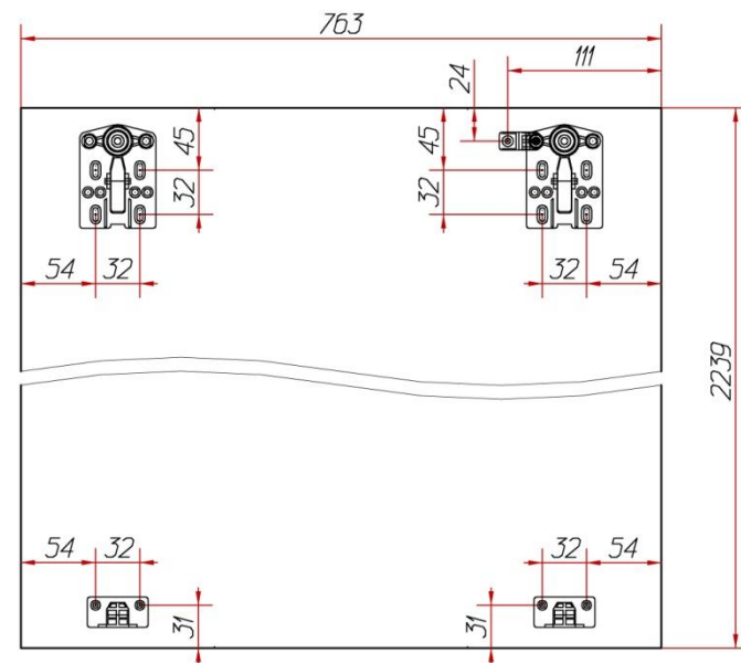
Дверь внутренняя:
