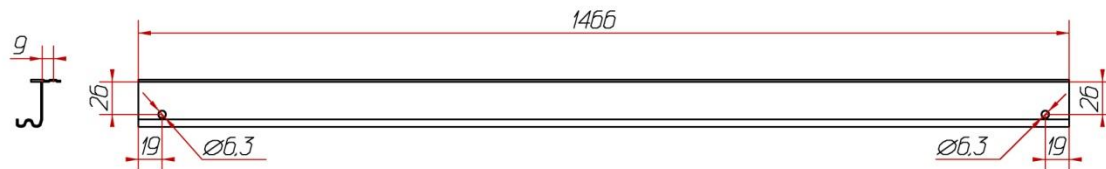
Ходовой профиль:
