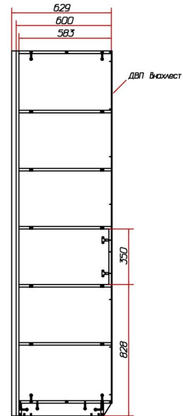
Вид справа:
