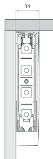
Вид спереди
