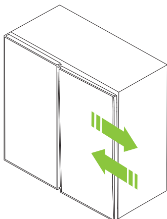
Бічне регулювання +2/-2 мм
