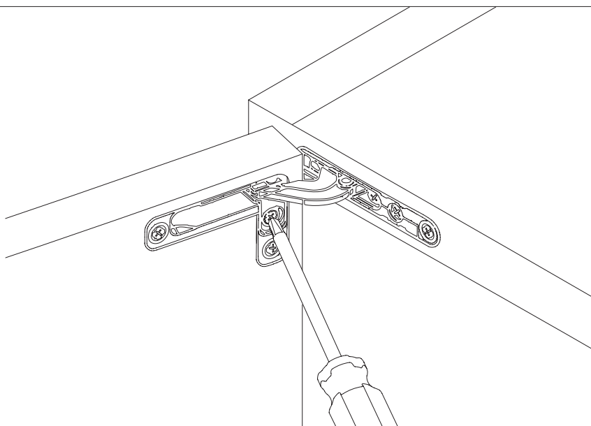
Регулювання по вертикалі +1,5/-1,5 мм
